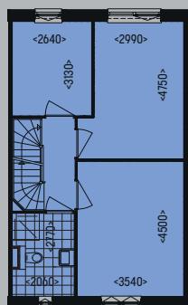
Eerste verdieping
