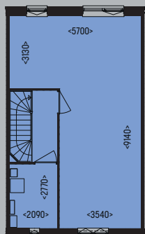
Tweede verdieping
